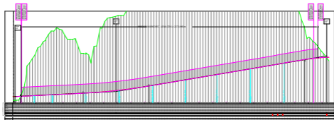
VZDOLŽNI PROFIL PREDORA MARKOVEC - LEVA CEV 1:5000
